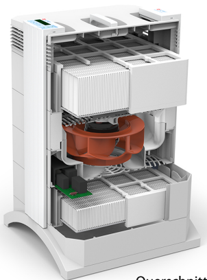
Querschnitt
